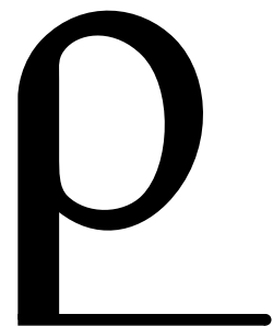
Pluto
