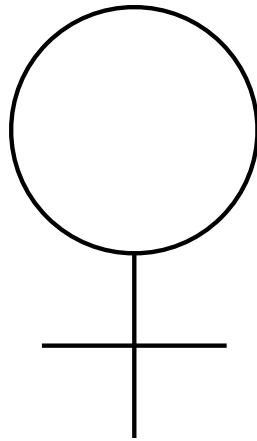
Venus
