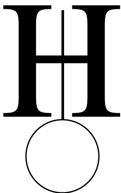
Uranus
