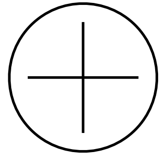
Earth
