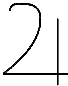
Jupiter
